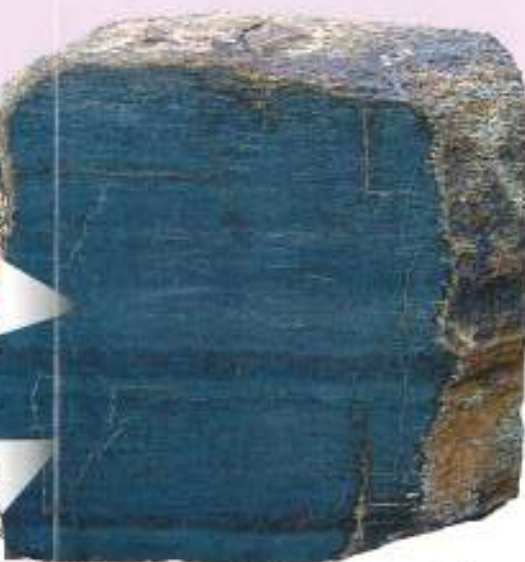
斜長石レゾライト (Plagioclase Lherzolite) は単斜輝石を多く含むかんらん岩で、多量のマグマを生成することができます。鉄やチタンに富むため、暗い紫色を呈します。平行な2枚の層は斜方輝石と単斜輝石からなる層岩 (さがん, Pyroxenite) です。
