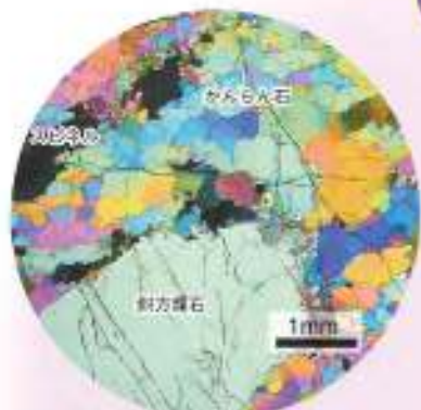
ハルツバージャイト (Harzburgite) の偏光顕微鏡写真。主にかんらん石と斜方輝石からなるかんらん岩です。マグマが抜け切った後の融け残りのかんらん岩です。
