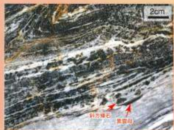
斜方輝石グラニュライト (Orthopyroxene Granulite) ミグマタイト質の岩石で、部分融解の過程を示しているかもしれません。
