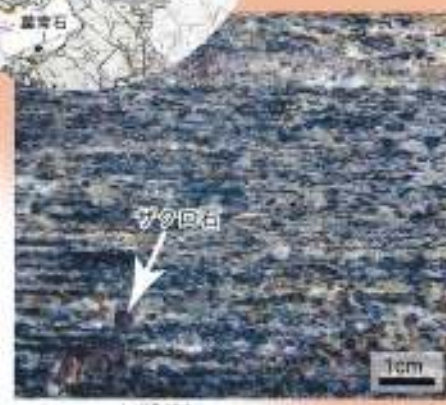
ザクロ石-斜方輝石グラニュライト (Garnet-Orthopyroxene Granulite) は非常に高温の変成作用を受けて出来た岩石で、下部地殻を構成する代表的な岩石です。
