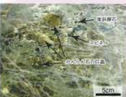
ダナイト (Dunite) は、かんらん石がほとんどを占めるかんらん岩です。マグマの通り道と考えられています。
